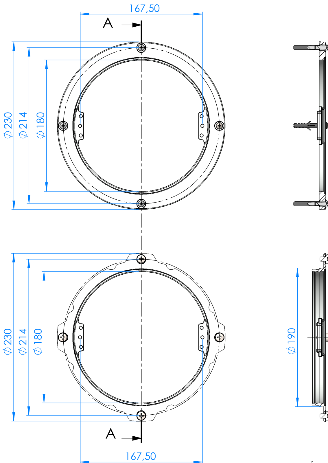
SECCIÓN A-A
