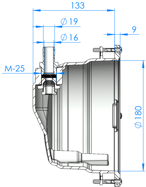
SECCIÓN A-A
